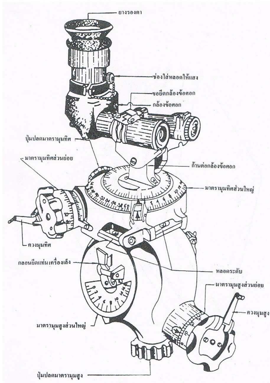
ภาพที่ 13 กล้องเล็งแบบ M53 A1
