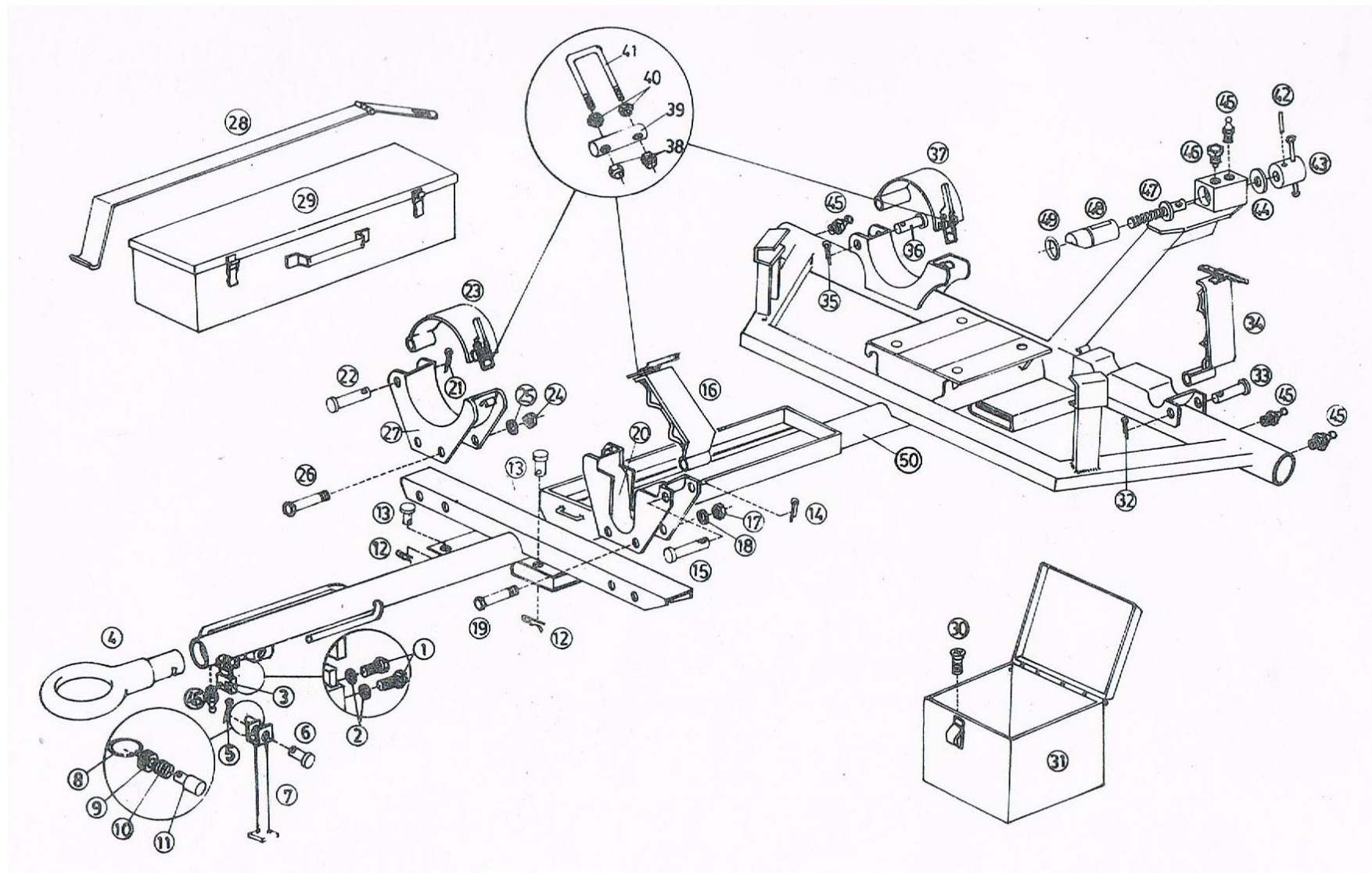
ภาพที่ 11 ชุดโครงรถ
