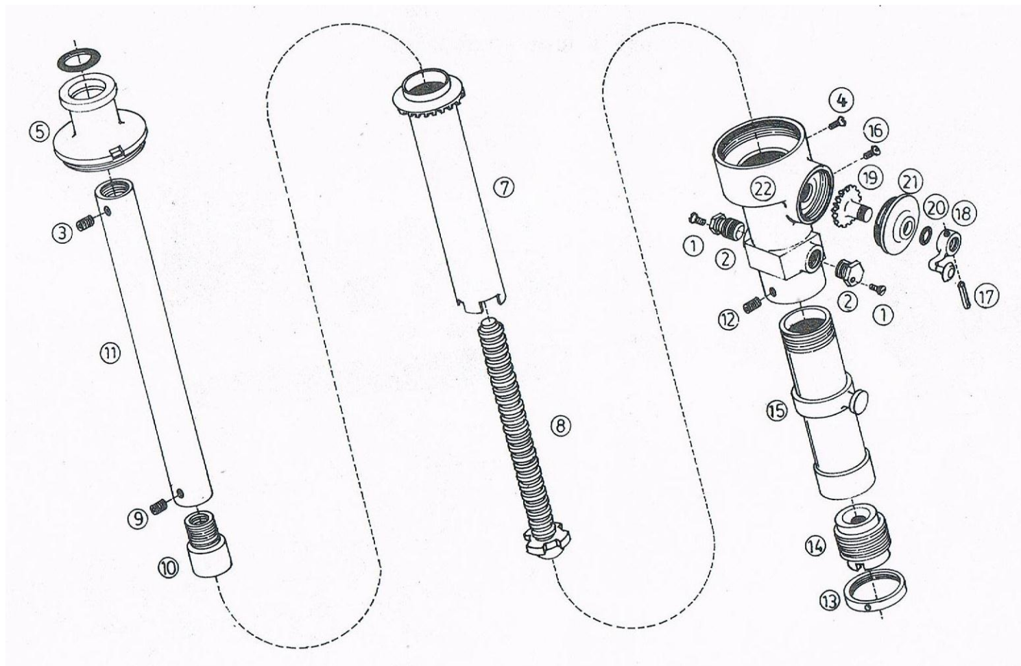
ภาพที่ 6 ชุดเครื่องให้มุมทางสูง
